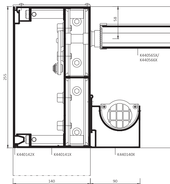
Řez prostřední krokví
