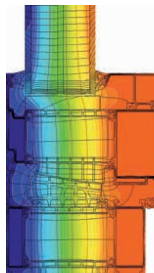
Rozložení izoterm v okně MB-104 Passive Aero
