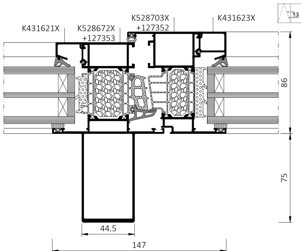
Okno MB-86N SI ve fasádě MB-SR50N
