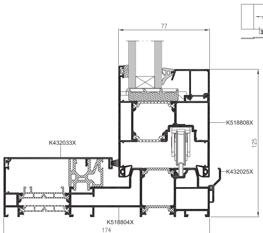
Spodní řez dveřmi s fixem
