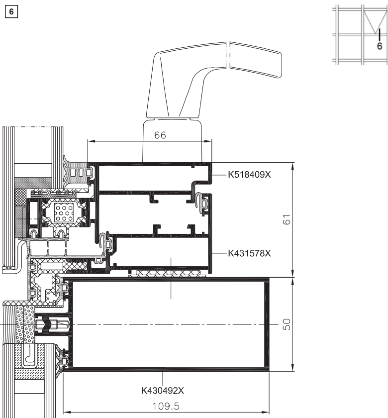
Řez fasádou s oknem ven výklopným MB-SR50N OW
