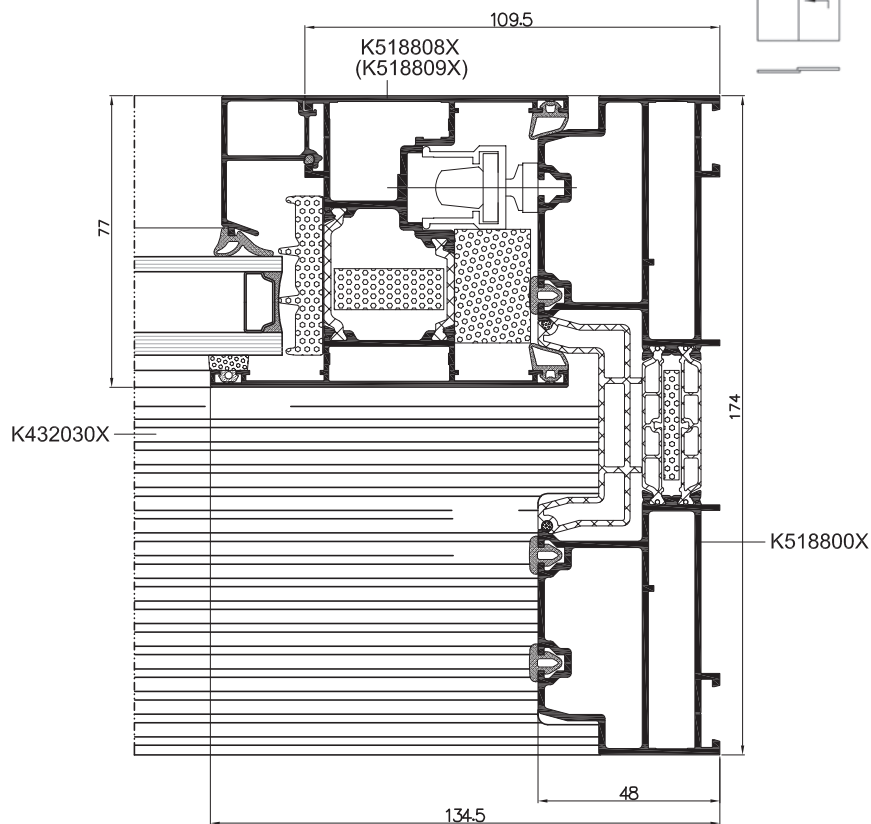
Boční řez dveřmi
