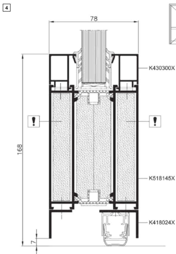
Řez prahem dveří s padacím prahem MB-78EI
