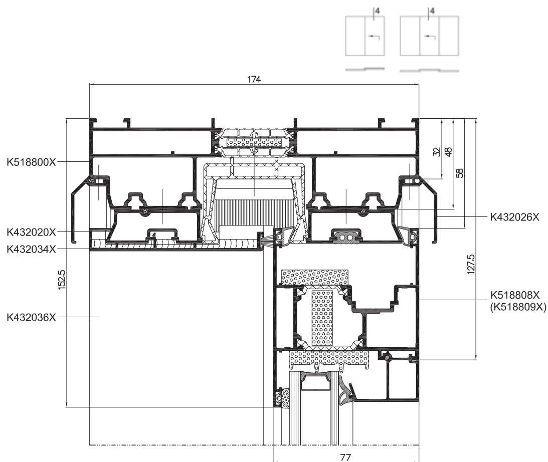
Spodní řez dveřmi
