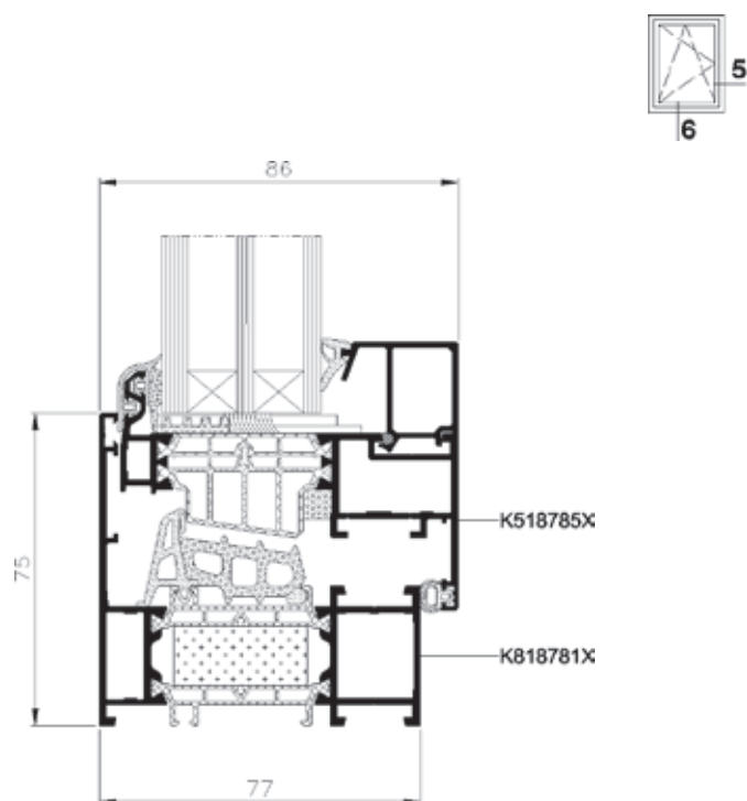
Řez otvíravým oknem MB-86US SI
