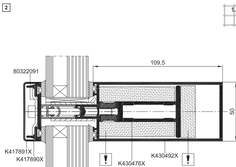
Řez příčným EI 15, EI 30
