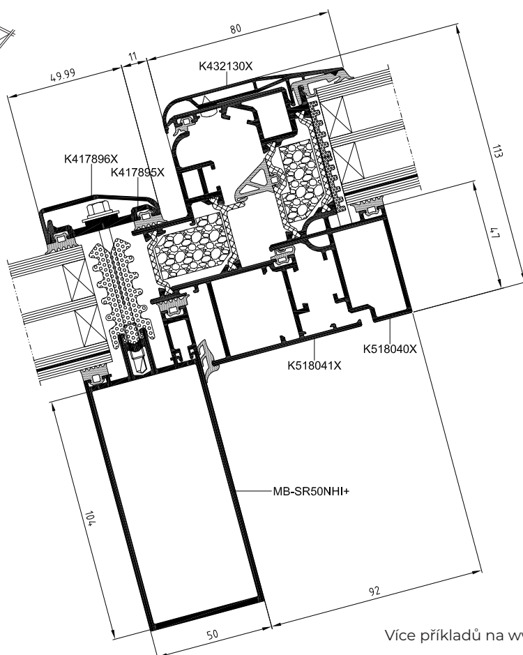
Řez střešním oknem MB-RW ve fasádě MB-SR50N HI+
