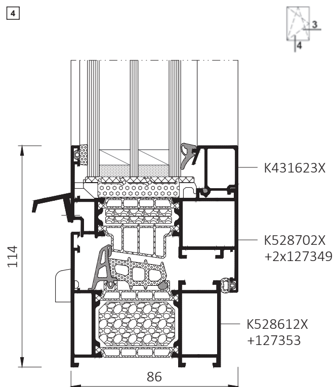
Řez otvíravým oknem MB-86N SI
