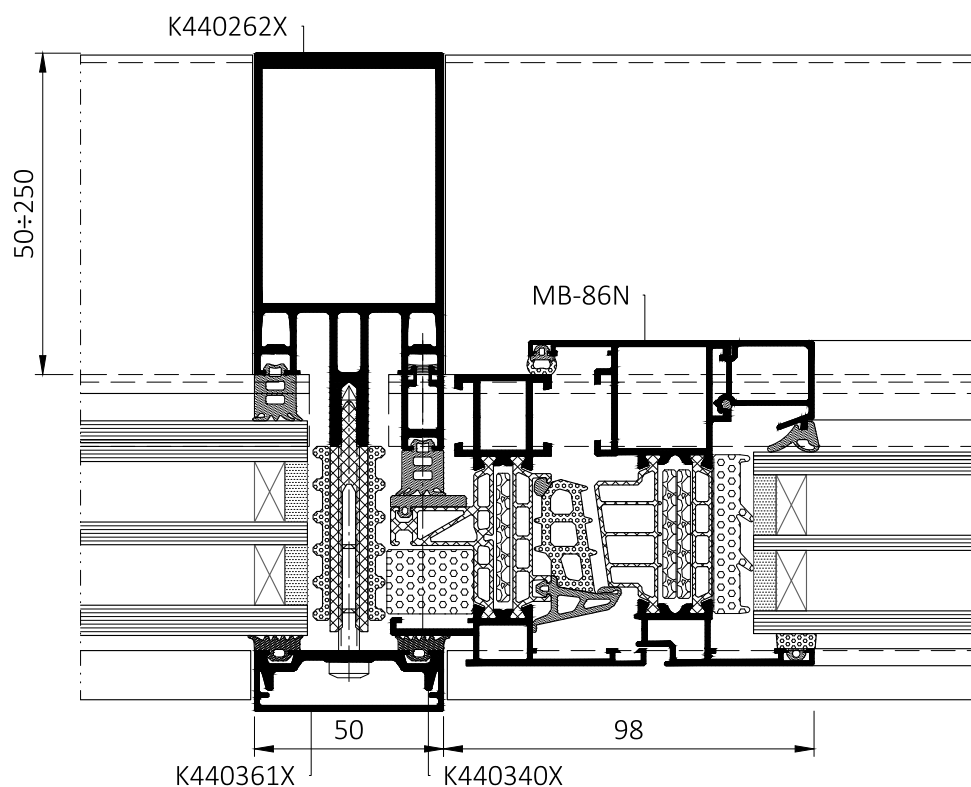
Řez sloupkem MB-MT50N SI a okna MB-86N
