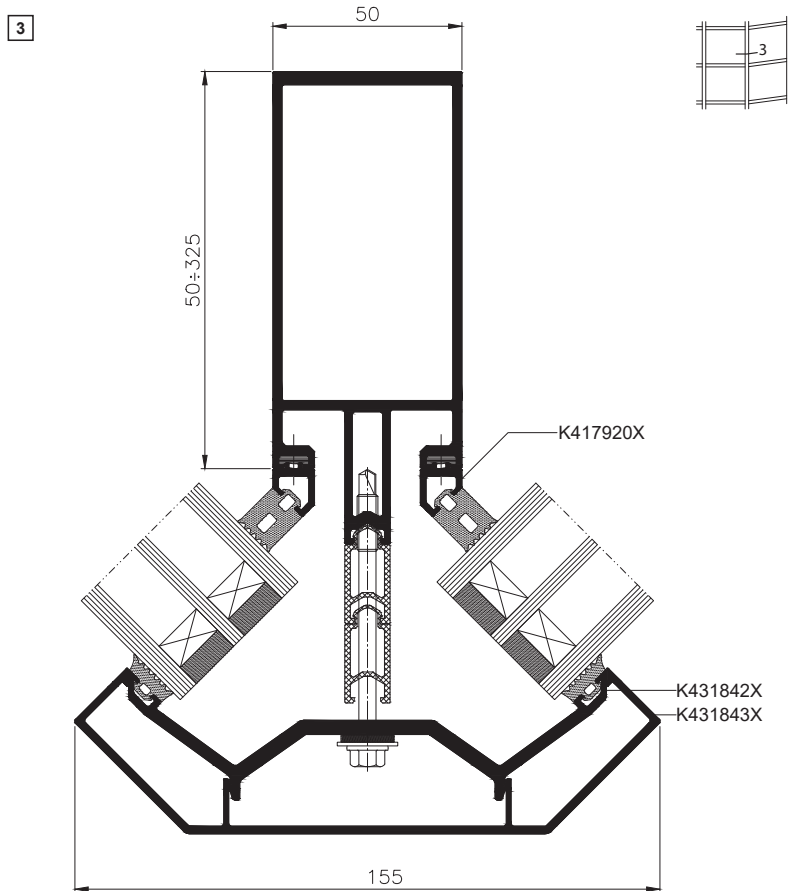
Řez úhlovým sloupem
