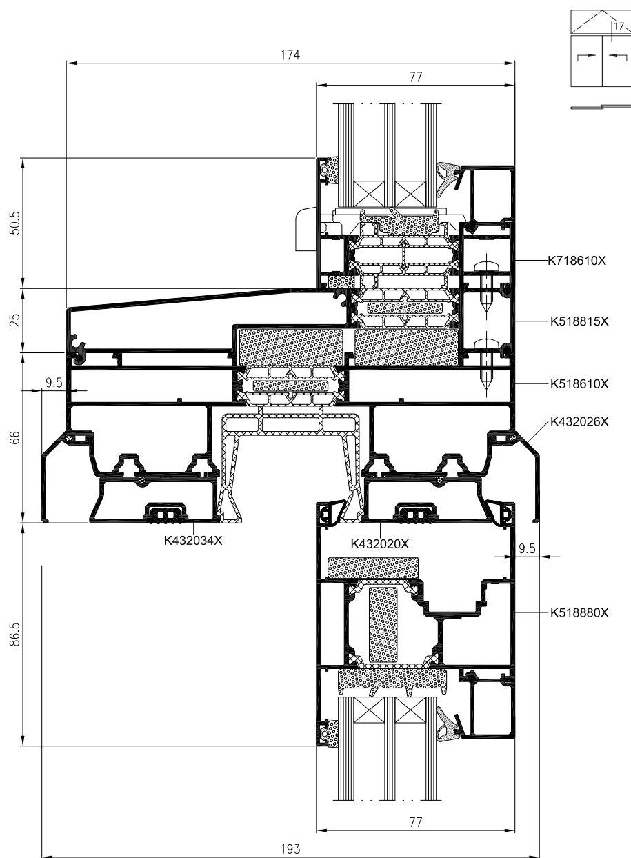
Řez dveřmi s nadsvětlíkem
