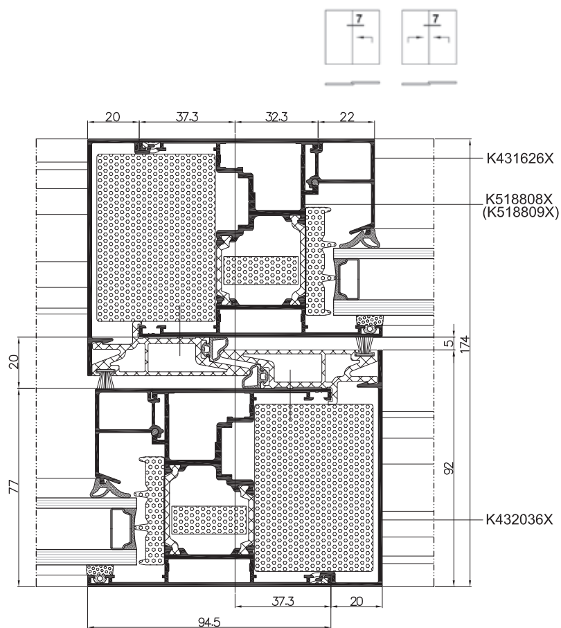
Řez křídly dveří
