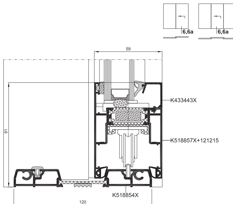
Dolní řez dveřmi s nízkým prahem
