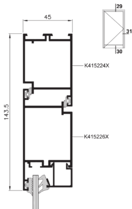
Dveře "Standard" – jednokřídlé otvíravé ven – řez
