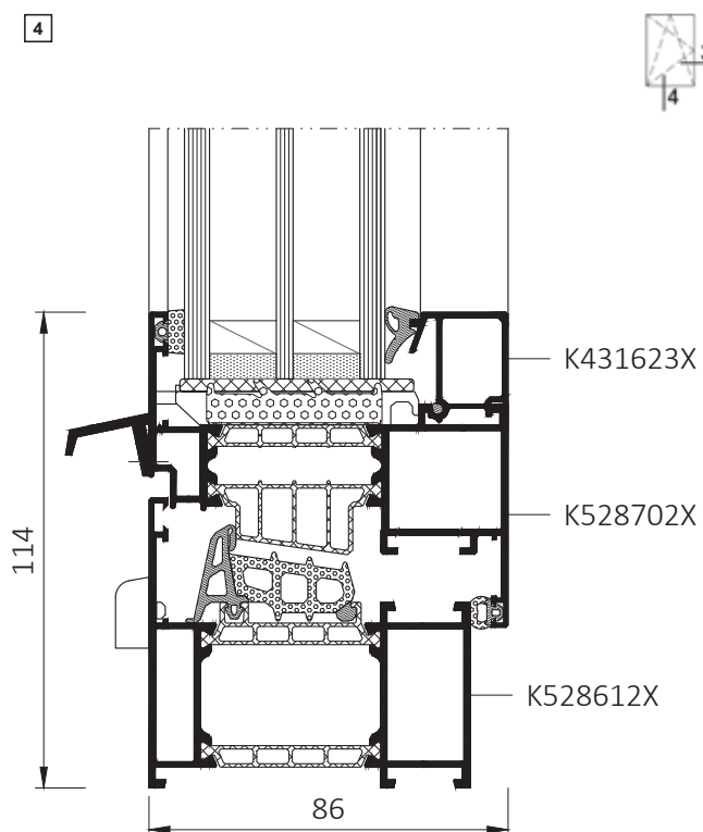
Řez otvíravým oknem MB-86N ST
