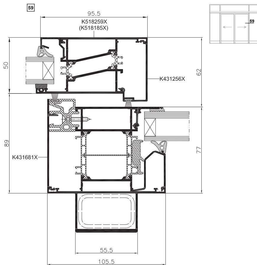
Dveře posuvné ve vitrině MB-86 – řez
