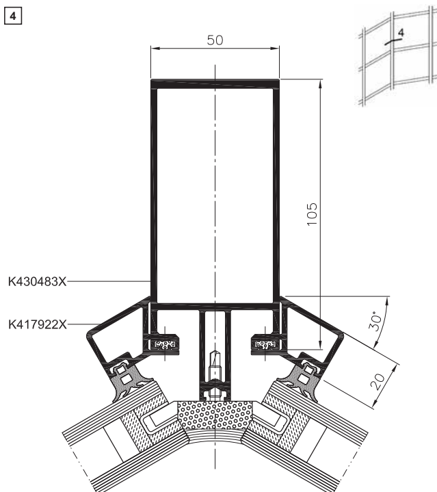
Řez úhlovým sloupem
