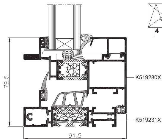
Řez otevíraným oknem - typ A
