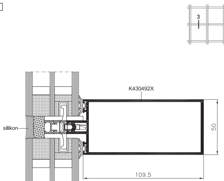
Řez příčkou
