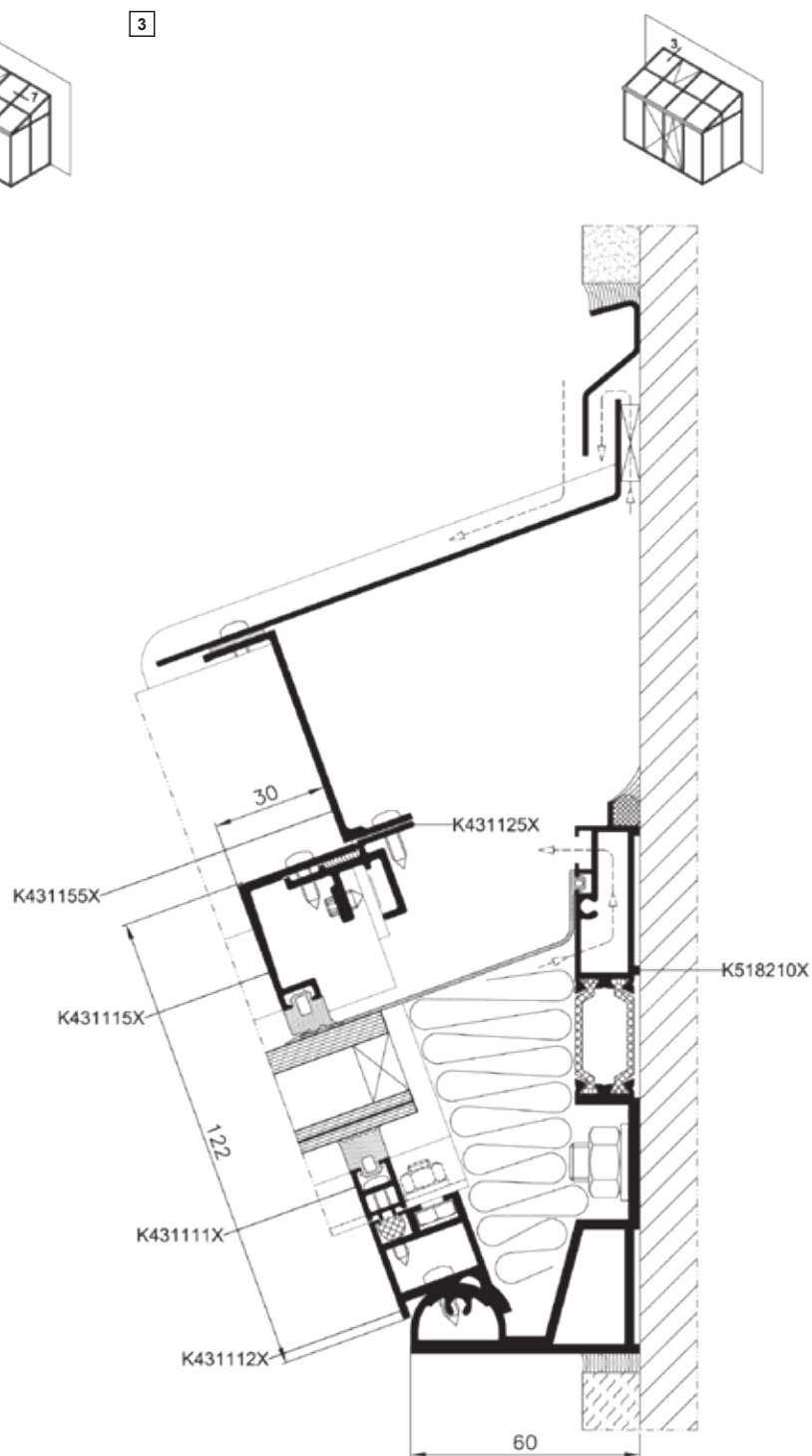
Řez příčkou
