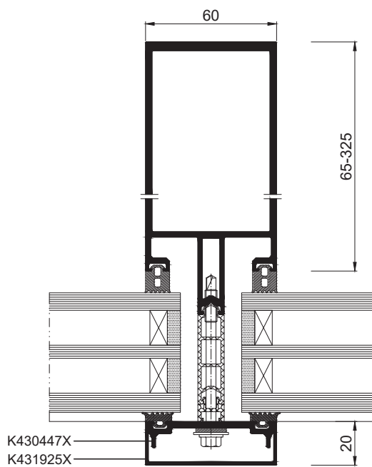
Řez sloupem
