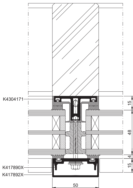
Řez sloupkem
