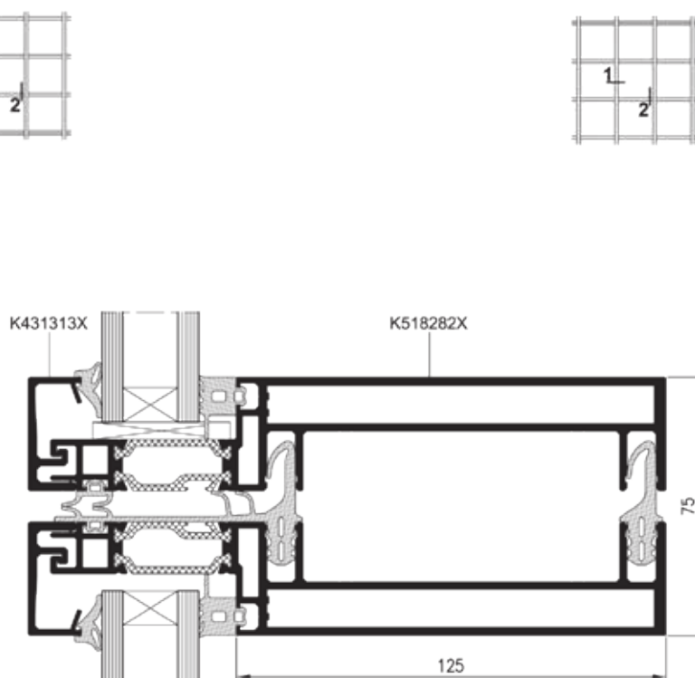
Řez příčkou
