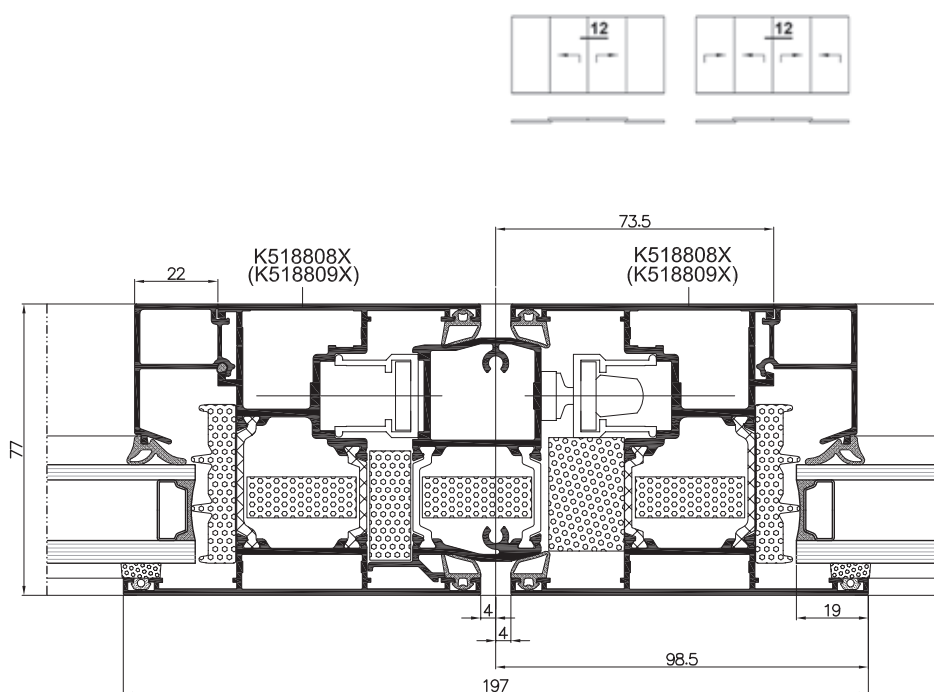
Řez křídly dveří
