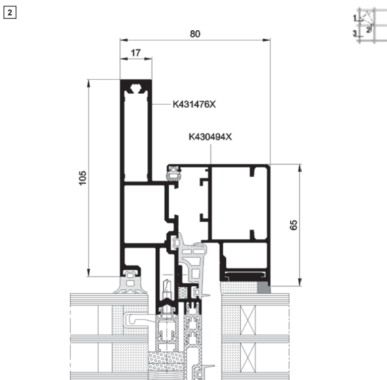
Řez sloupkem - verze EFEKT
