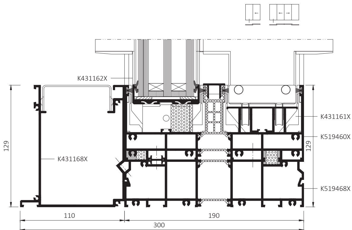
Dolní řez kolejnicí MB-SKYLINE TYPE R
