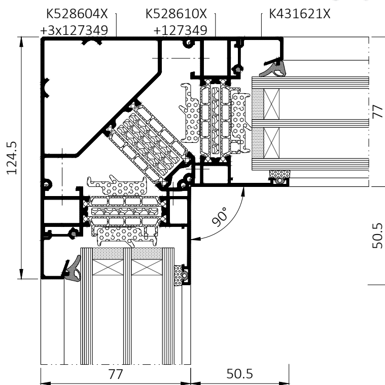
Řez úhlovým spojením MB-86N SI
