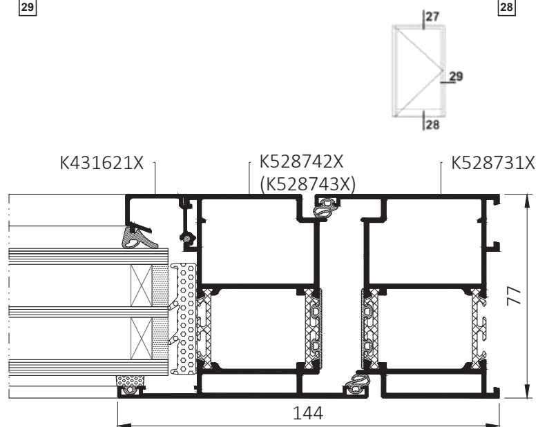
Řez dveřmi MB-86N ST
