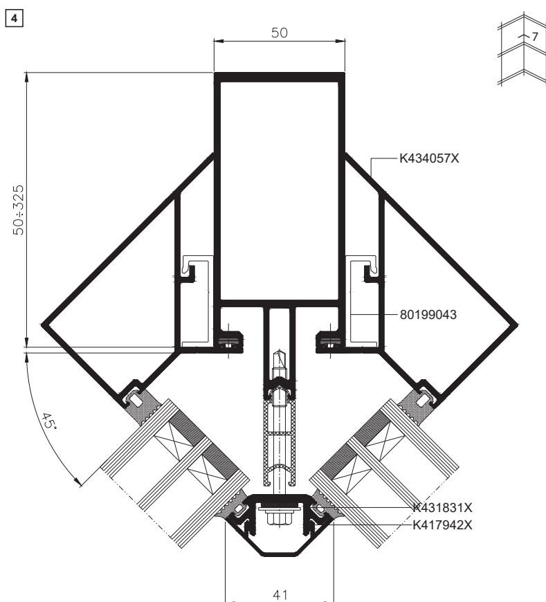
Řez úhlovým sloupem
