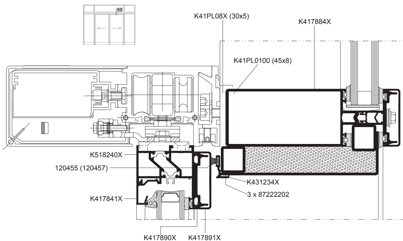
Dveře posuvné ve fasádě MB-SR50N – řez
