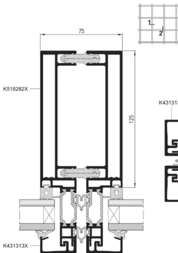
Řez sloupem
