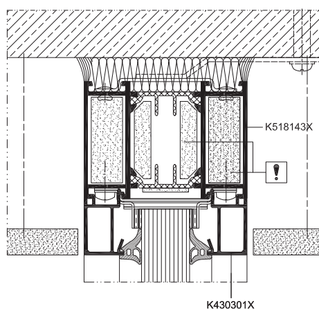
Řez stěnou s profilem zabudovaným v podlaze
