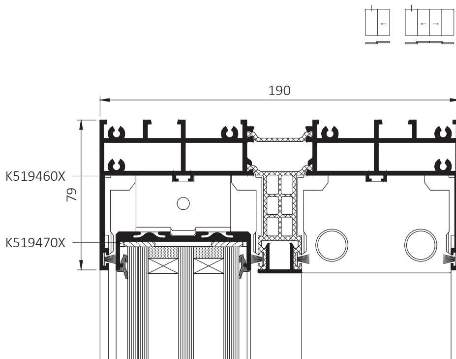
Horní řez kolejnicí MB-SKYLINE TYPE R
