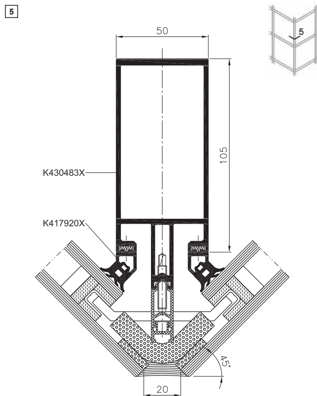
Řez úhlovým sloupem
