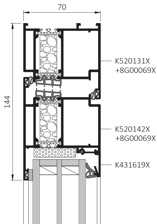
Řez dveřmi MB-79N SI+
