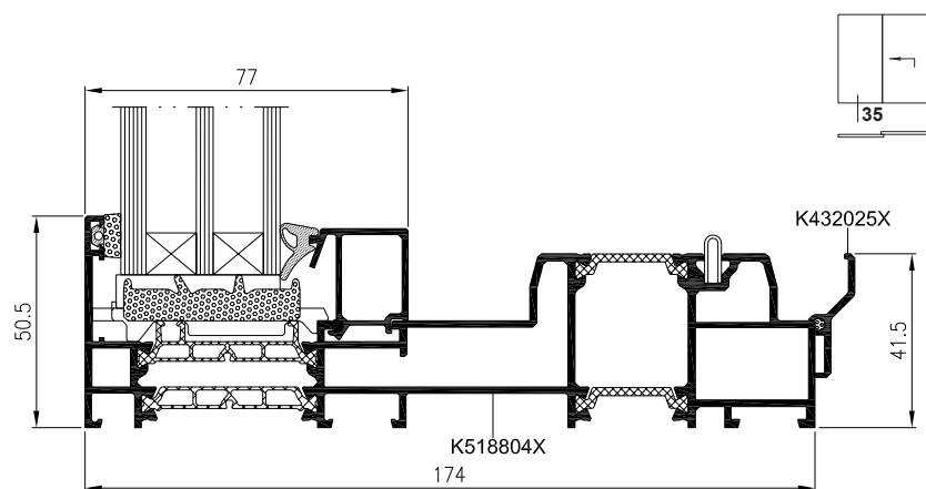
Spodní řez dveřmi s pevným oknem
