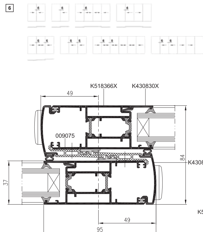
Řez svislými profily křídel
