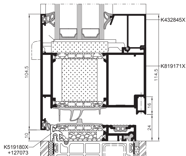
Řez prahem dveří MB-104 Passive AERO
