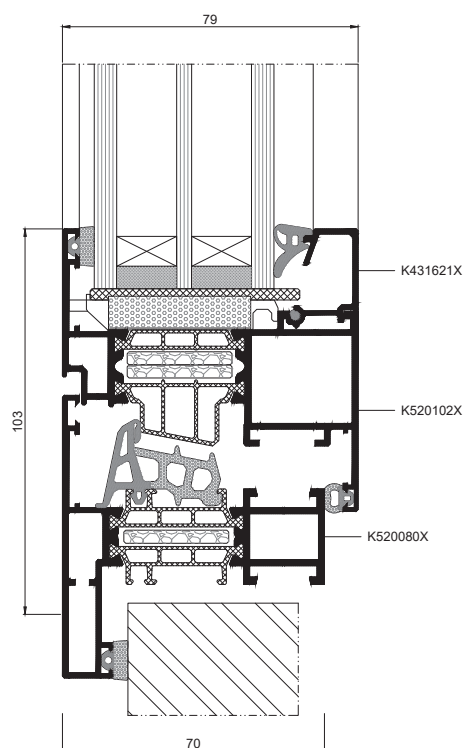
Řez otvíravým oknem MB-79N SI s překryvným rámem
