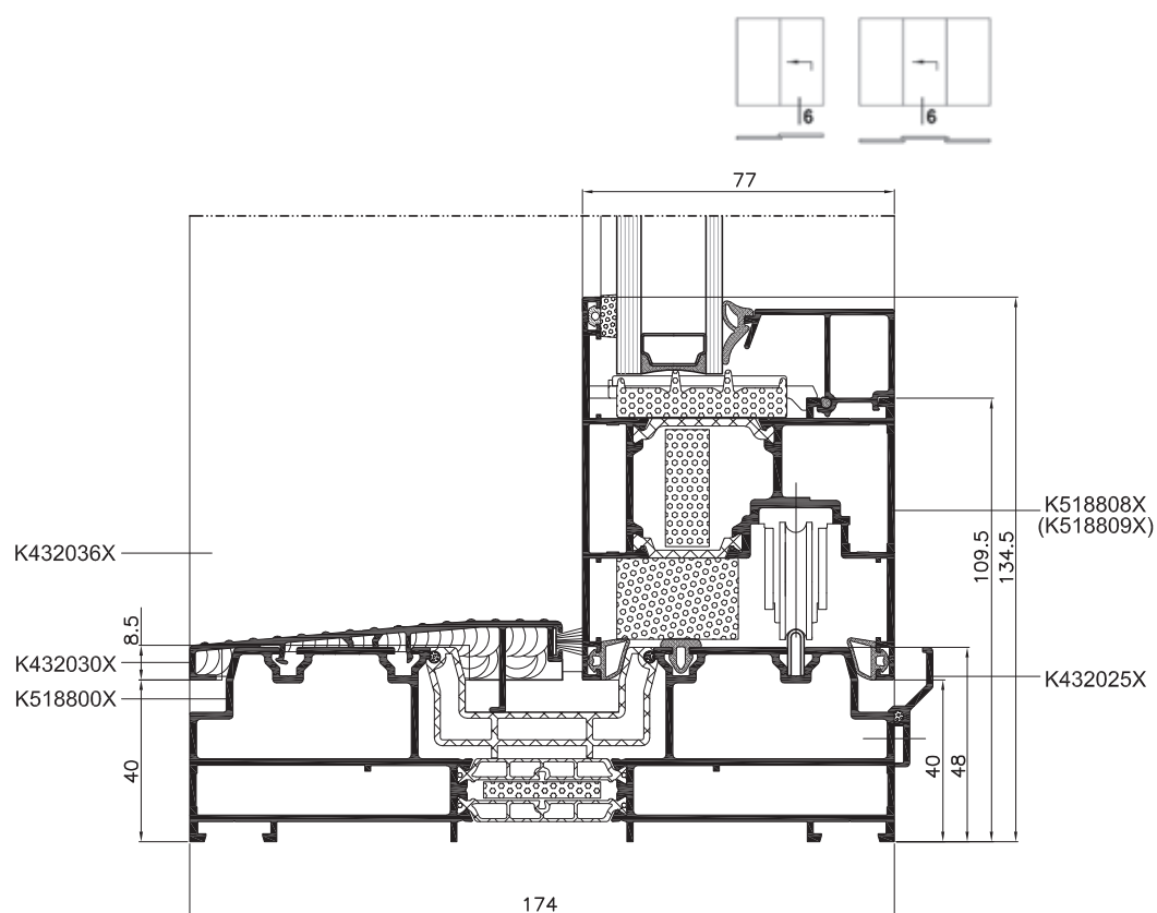
Spodní řez dveřmi
