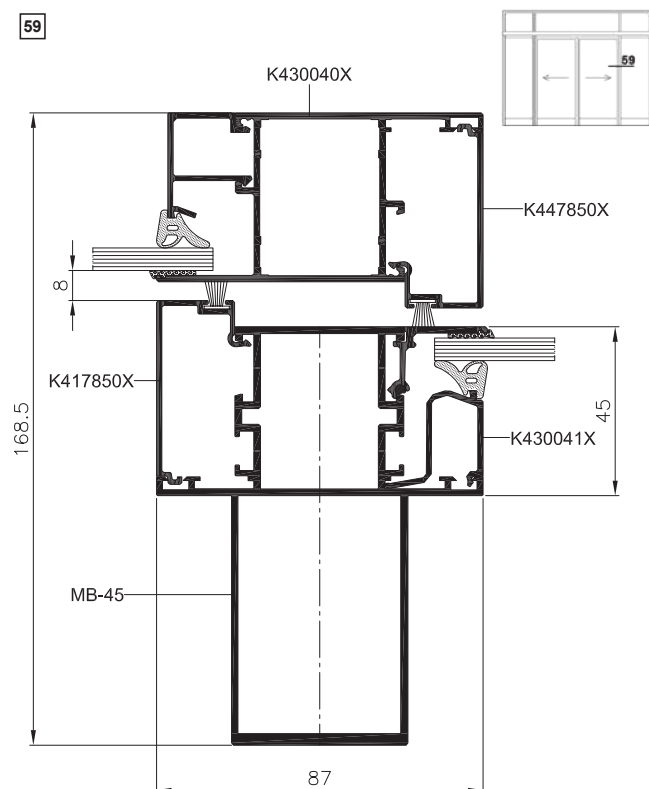
Dveře posuvné – řez
