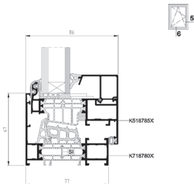
Řez otvíravým oknem MB-86US ST
