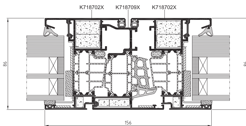
Řez 2kř. oknem MB-86EI
