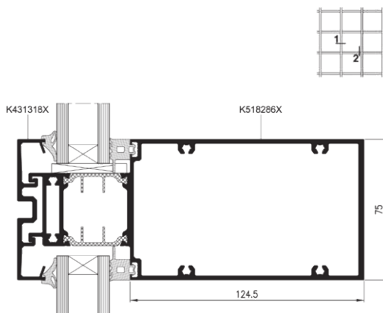
Řez příčkou
