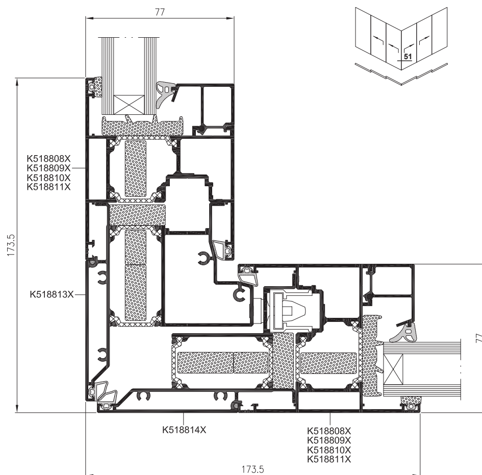
Řez otvíravým rohovým spojením (vnějším)
