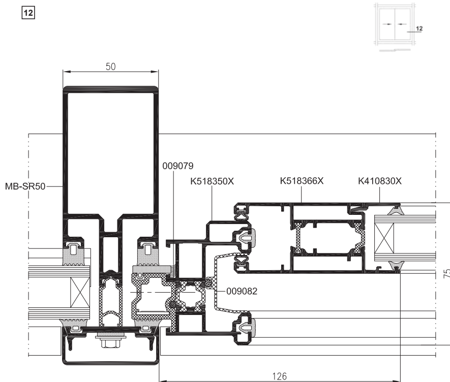
Řez dveřmi ve fasádě MB-SR50N
