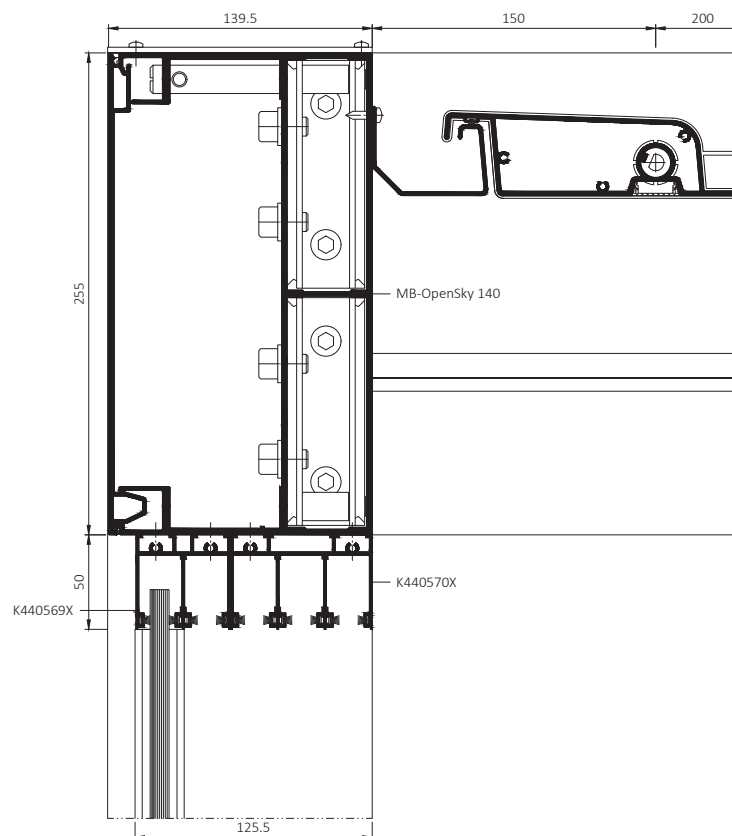
Řez krokví pergoly a horního vedení MB-Open Slide
