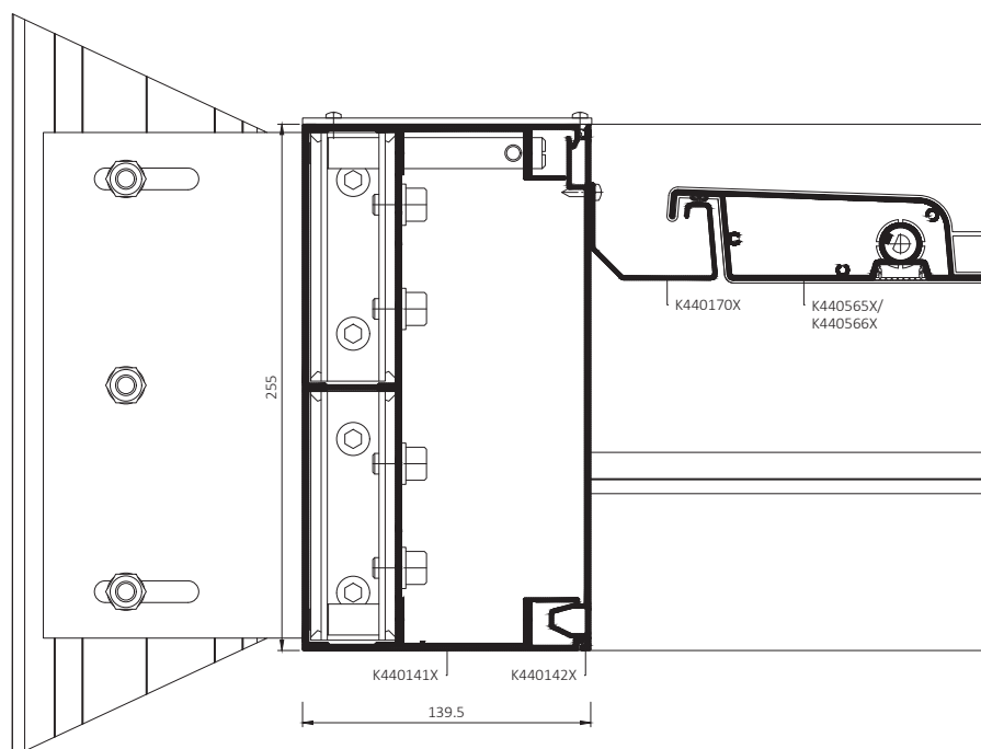
Řez krokví napojenou na zeď
