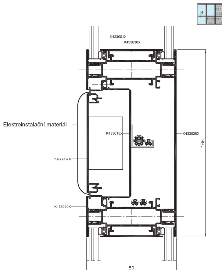
Svislý řez příčkou s elektroinstalačním materiálem
