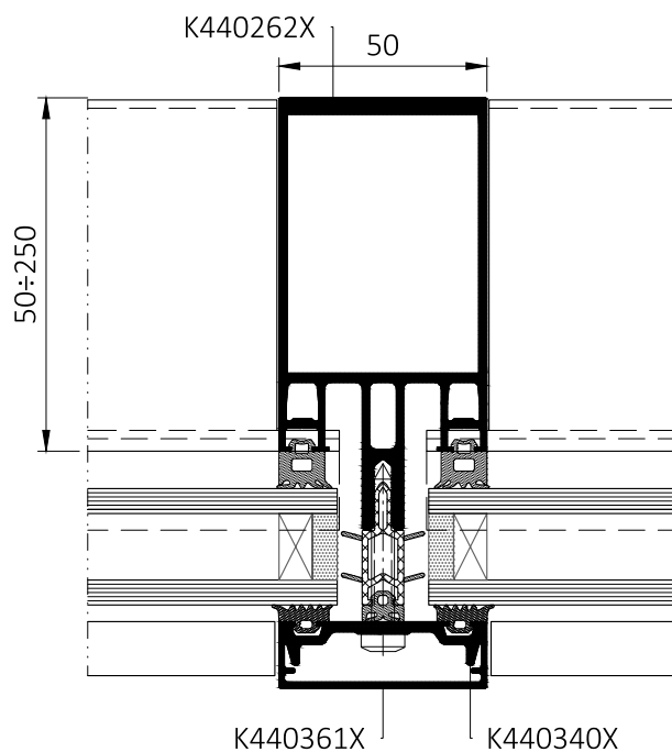
Řez sloupkem MB-MT50N
