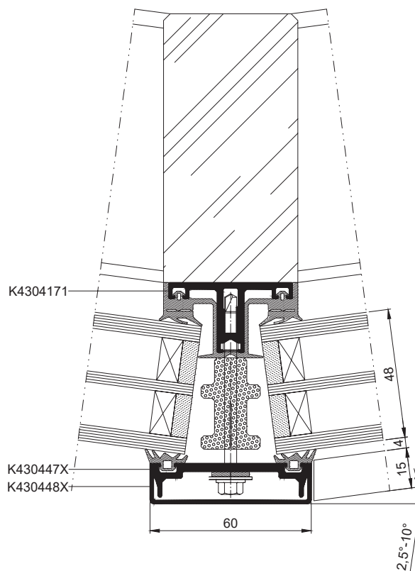
Řez příčkou
