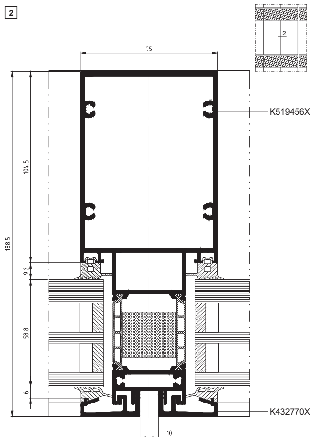
Řez sloupem
