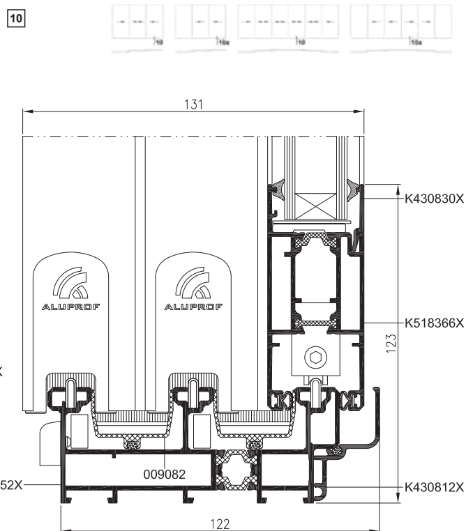
Řez spodní příčkou dveří
