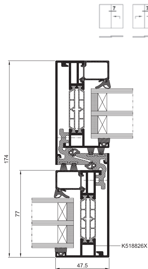
Řez úzkými křídly
