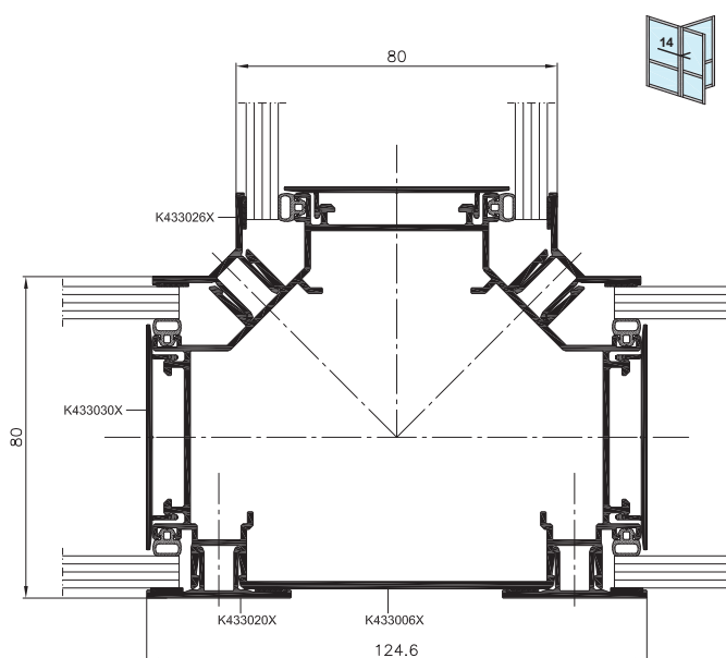
Řez spojem tří stěn
