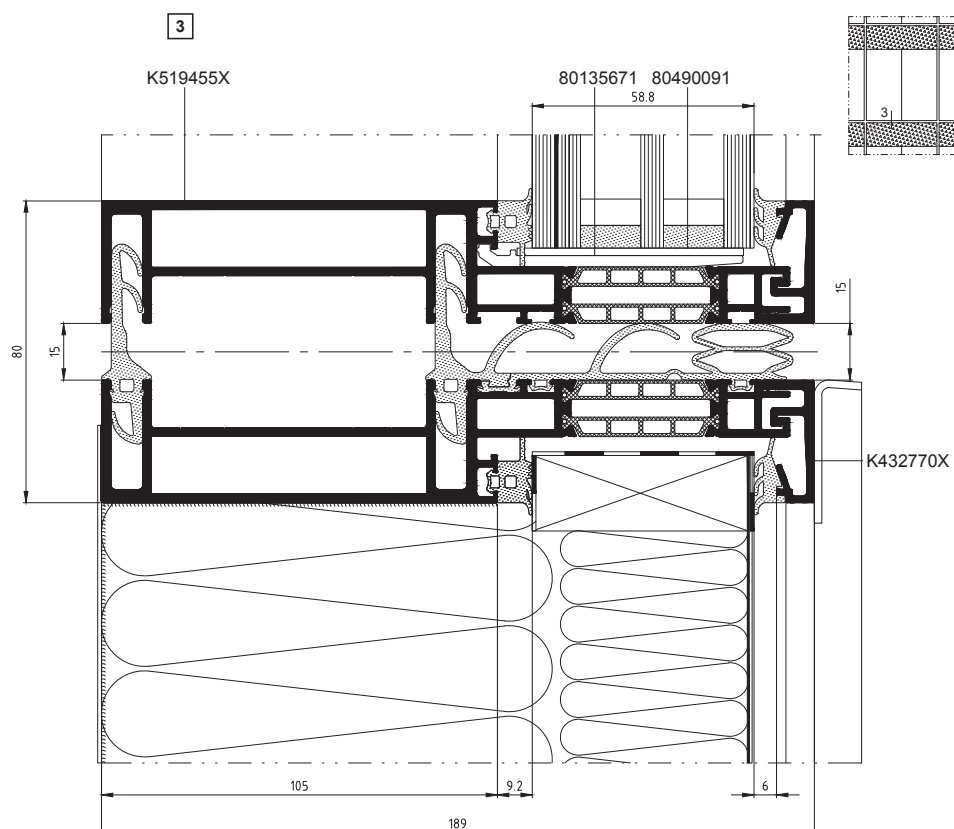
Řez příčkou
