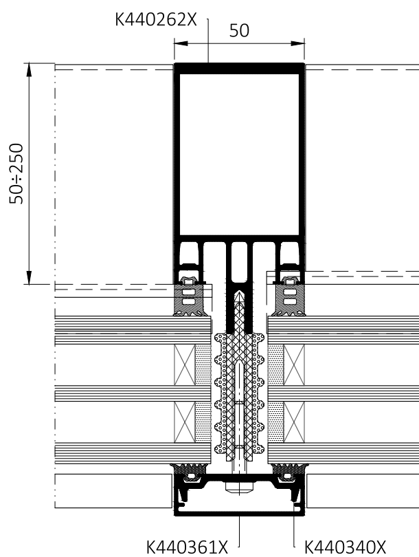
Řez sloupkem MB-MT50N SI
