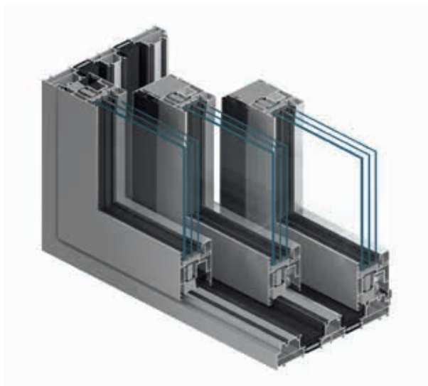
3kolejnicový rám
