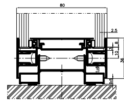
Schnitt durch das untere Basisprofil
