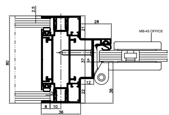
Türschnitt
