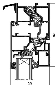
Nach außen öffnende Fenster – Schnitt
