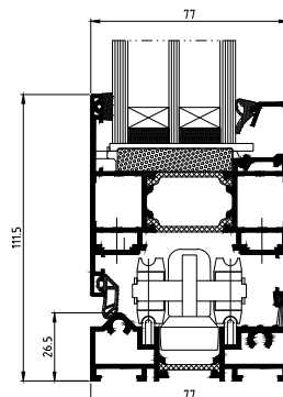
Unterer Schnitt Tür mit niedriger Schwelle
