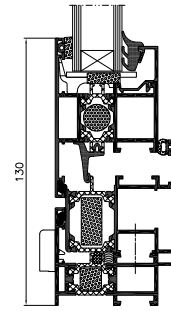
Schwingflügel Fenster – Schnitt
