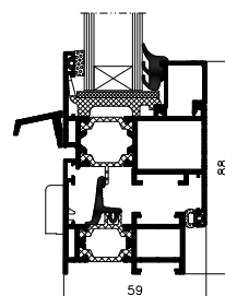
Stulpfenster – Schnitt
