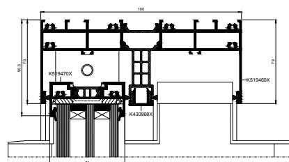
Schnitt Türoberseite
