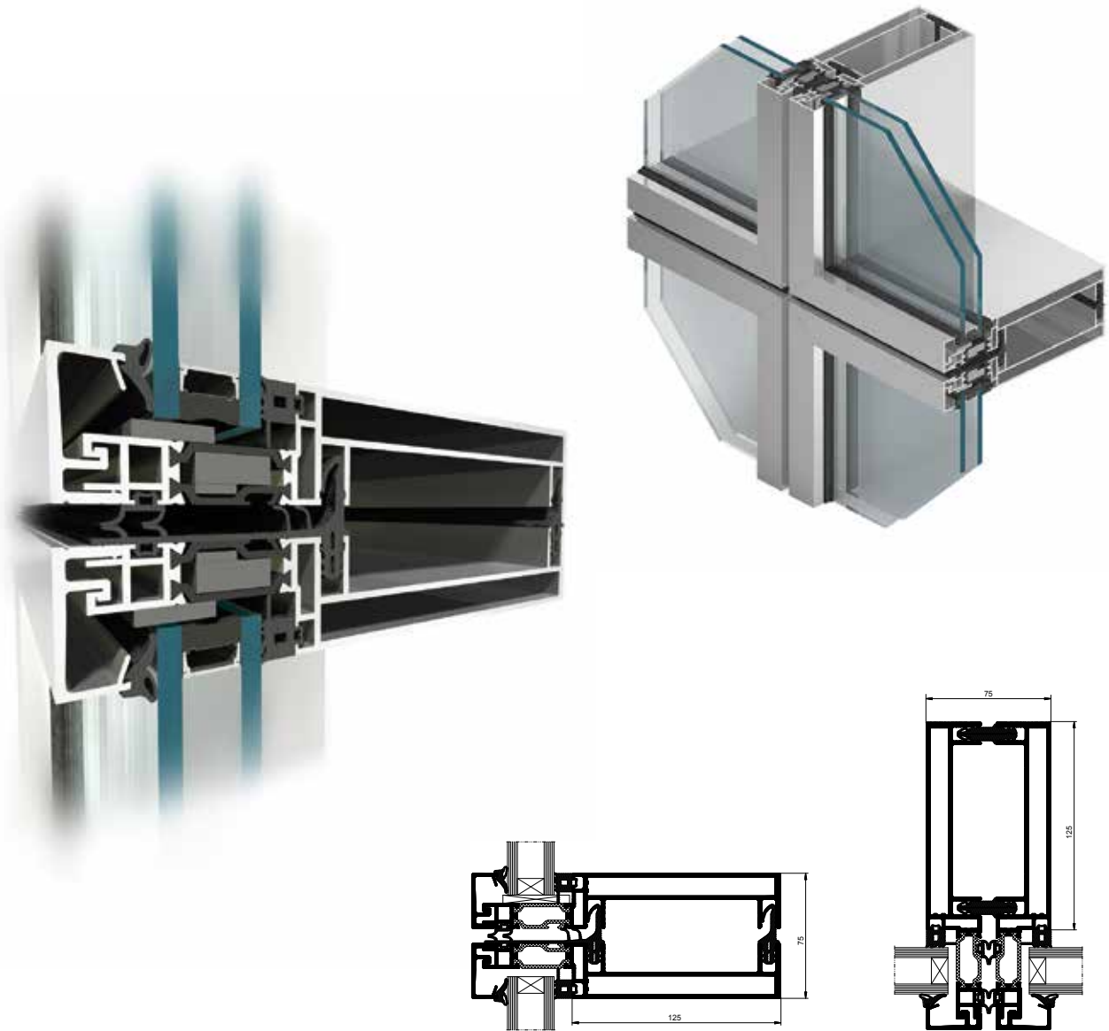
Riegel – Schnitt
