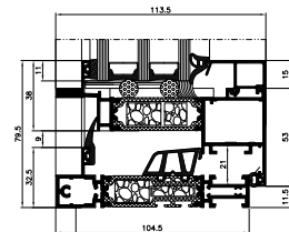
Schnitt durch das Fenster
