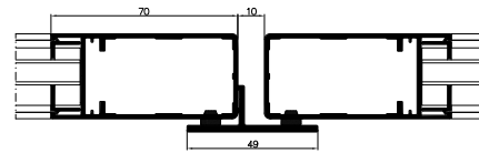
Waagerechter Schnitt durch den Flügel
