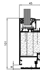
Tür – Schnitt
