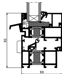
Fenster – Schnitt
