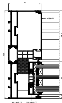
Seitlicher Schnitt der Tür
