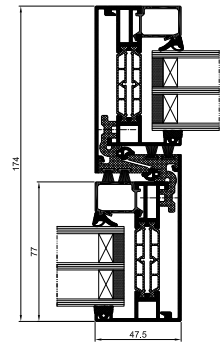
Stulpschnitt
