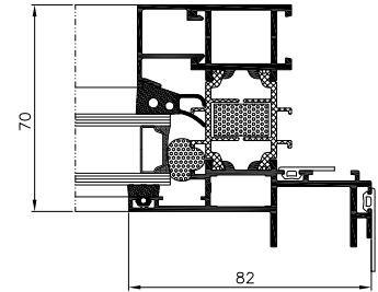
Schnitte durch Fenster MB-70US
