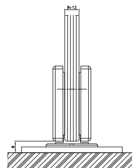
Schnitt des Schaufensters
