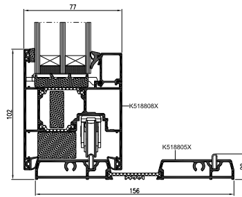
Unterer Schnitt Tür mit niedriger Schwelle
