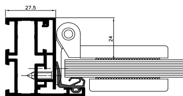
Seitlicher Türschnitt
