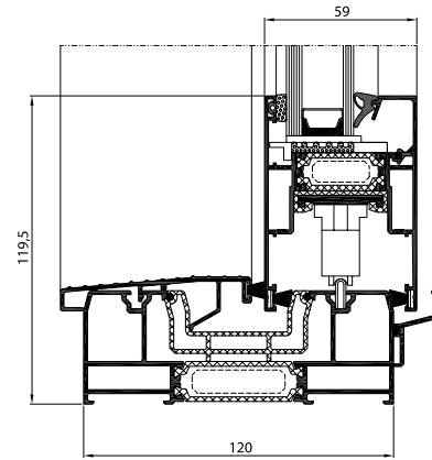
Schnitt durch Tür mit Blendrahmen mit einer Laufschiene
