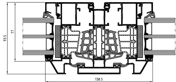
Schnitt durch Pfosten und Fenster
