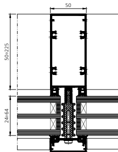
Schnittansicht eines Pfostens
