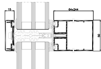
Riegel – Schnitt
