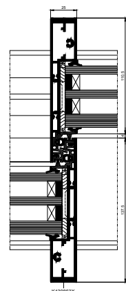
Schnitt durch die Flügel-Tür Verbindung
