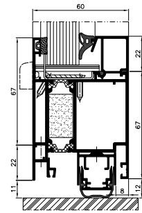
Schnitt durch Tür EI30
