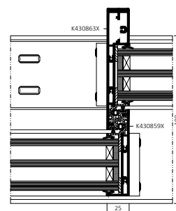
Schnitt durch die Türflügelverbindung
