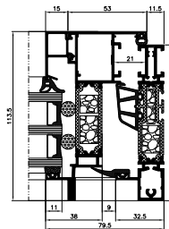
Schnitt durch das Fenster
