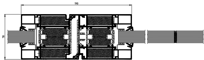
Schnitt durch Tür EI30
