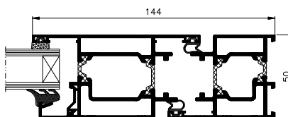
Tür – Schnitt
