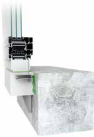
Verbindung unten, 100 mm Träger mit Außenanker
