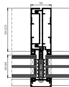
Schnittansicht eines Halbpfostens
