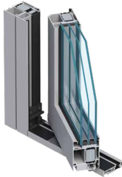
Glastür MB-86N PIVOT DOOR
