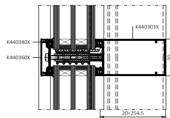
Schnitt durch den Riegel der 1. Reihe MB-MT50N SI
