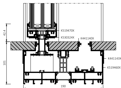
Schnitt Türunterseite
