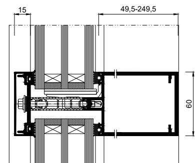
Riegel – Schnitt
