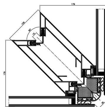
Schnitt durch den Eckpfosten
