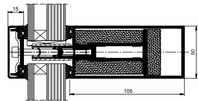
Riegel – Schnitt EI 15, EI 30
