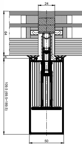
Pfosten – Schnitt EI 45, EI 60
