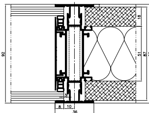
Schnitt durch Wand 92 mm
