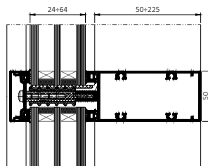
Schnittansicht eines Riegels
