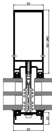
Pfosten – Schnitt
