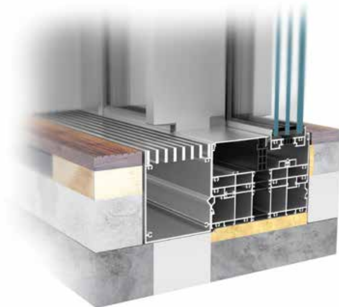
Seitlicher Blendrahmenschnitt
