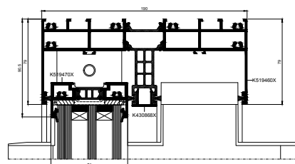
Boven doorsnede van de deur
