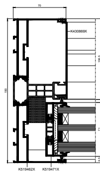
Dwarsdoorsnede zijkant deur
