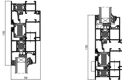
dwarsdoorsnede pivotraam
