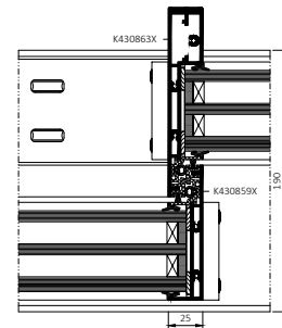
dwarsdoorsnede van de vleugelverbinding van de deur
