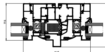
dwarsdoorsnede opengaand en vast raam
