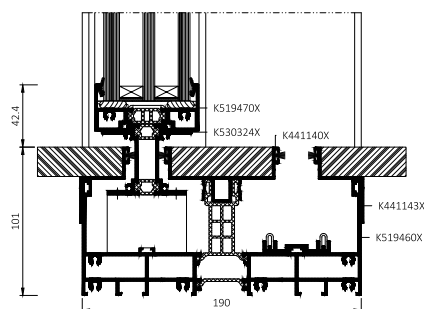
Onder doorsnede van de deur
