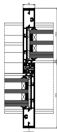
Doorsnede van de vleugelverbinding van de deur
