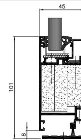
dwarsdoorsnede deur
