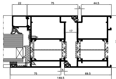
onderste doorsnede van een deur EI30
