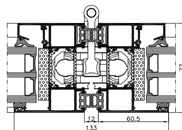
dwarsdoorsnede door de verbinding van de deurvleugels
