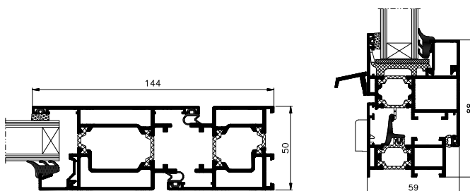
dwarsdoorsnede deur
