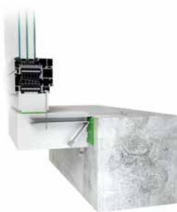
verbinding onder, op een balk van 200 mm met interne verankering
