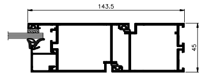
dwarsdoorsnede deur
