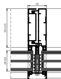
Sectie van een halve middenstijl
