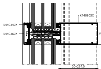
Dwarsdoorsnede door de dwarsbalk 1e rij MB-MT50N SI
