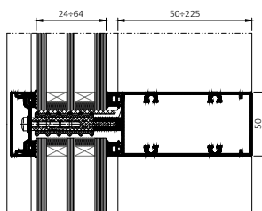
Sectie van een bovendorpel
