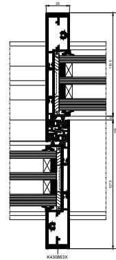
dwarsdoorsnede door de verbinding van de deurvleugels
