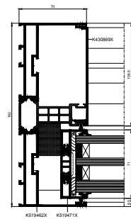
Dwarsdoorsnede zijkant deur
