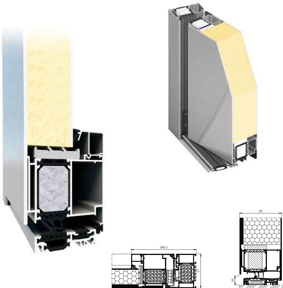
dwarsdoorsnede door de MB-86N SI+ paneeldeur
