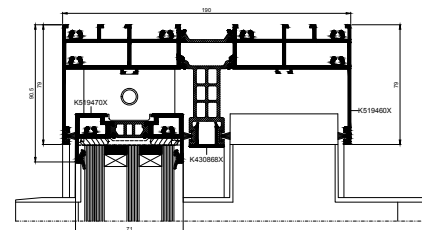
przekrój górny drzwi
