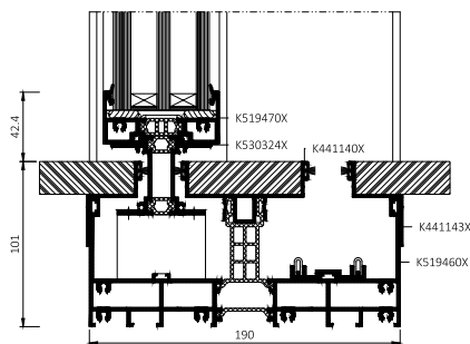
przekrój dolny drzwi
