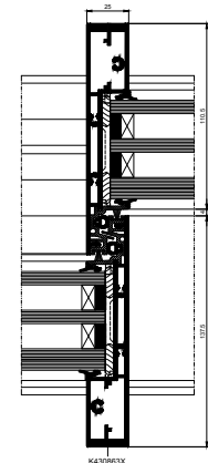
przekrój przez połączenie skrzydeł drzwi
