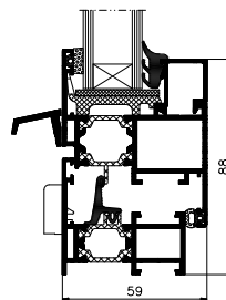
przekrój okna otwieranego
