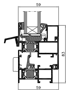
przekrój okna otwieranego
