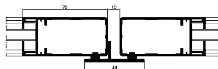
przekrój poziomy skrzydła z przylgą
