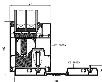
нижній переріз дверей з низьким порогом
