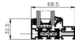
переріз по глухому вікну
