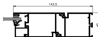
переріз по дверях
