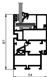
переріз по вікну
