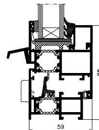
переріз відкривного вікна
