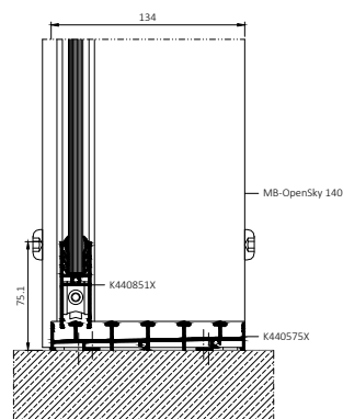
Поперечний розріз через ступку і поріг конструкції MB-OpenSlide
