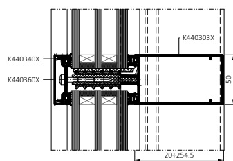
Розріз ригеля 1-го ряду MB-MT50N SI
