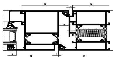
переріз дверей
