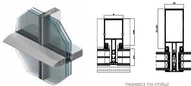
переріз по стійці
