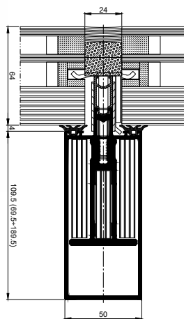
переріз по стійці EI 45, EI 60
