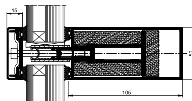
переріз по ригелю EI 15, EI 30
