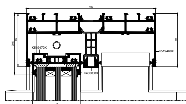
верхній переріз дверей
