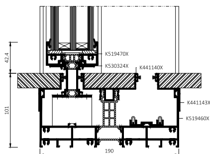
нижній переріз дверей
