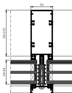
Розріз стійки
