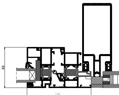
переріз по відкривному вікну в фасаді
