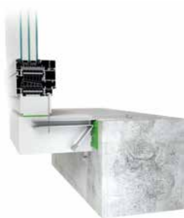
верхнє з'єднання із паронепроникною стрічкою та клеєм-ущільнювачем
