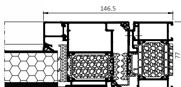
переріз по панельних дверях MB-86N SI+ у вітринній забудові
