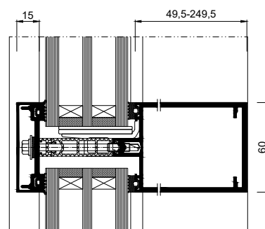
переріз по ригелю
