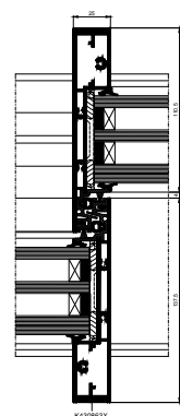
переріз з'єднання стулків дверей
