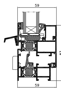
переріз відкривного вікна
