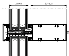
Розріз ригеля
