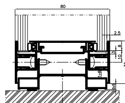
вертикальний переріз по стінці 92 мм
