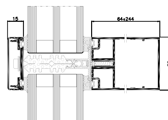
переріз по ригелю
