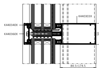
Розріз ригеля 2-го ряду MB-MT50N SI
