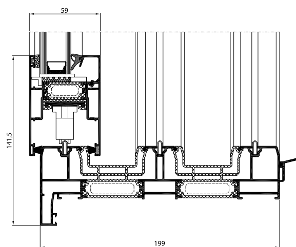
переріз дверей з 3-шинною коробкою
