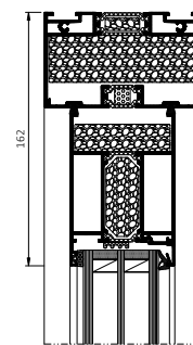
Верхній розріз дверей
