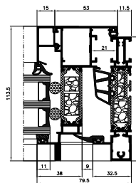
переріз по відкритому і глухому вікну
