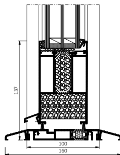
Розріз через дверний поріг
