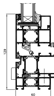
переріз по поворотному вікну
