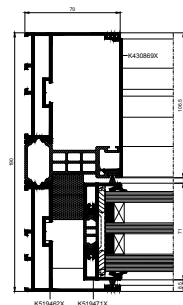
бічний переріз дверей
