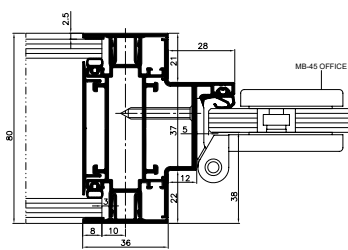
горизонтальний переріз дверей
