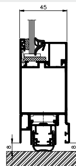
переріз по дверях
