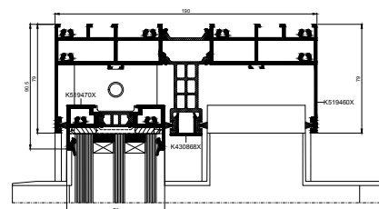
верхній переріз дверей
