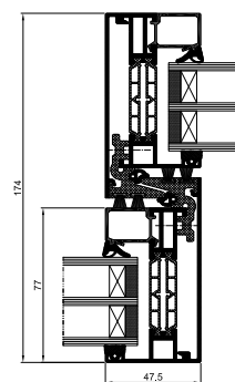
переріз по ступці дверей
