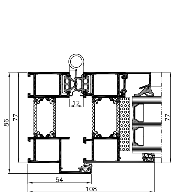
бокове сечение дверей
