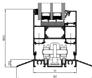
нижній переріз дверей з низьким порогом
